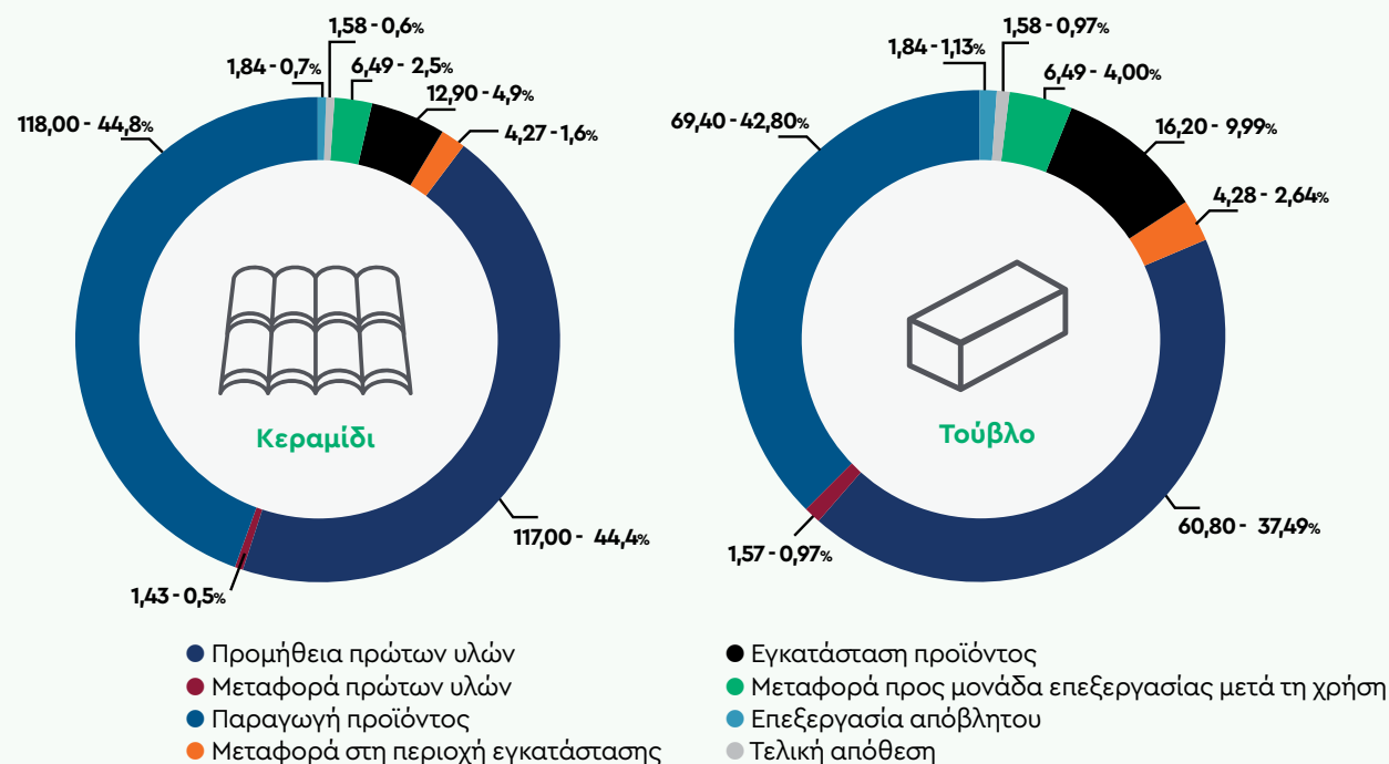
Ανθρακικό Αποτύπωμα Κεραμιδιού και Τούβλου σε kg CO 2 e ανά τόνο Προϊόντος
